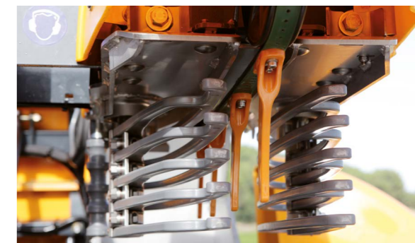
Égreneur linéaire cinq doigts
